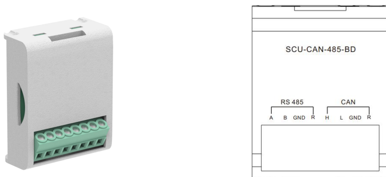
图 5-5 产品外观及端子定义
