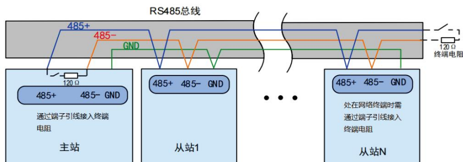
图 6-3 RS485总线通信连接
