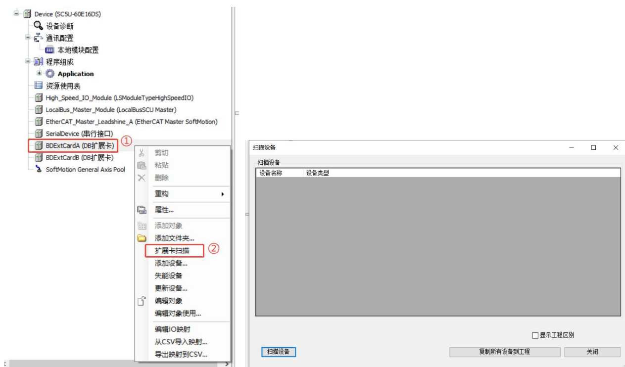
图 5-1通过“扩展卡扫描”方式添加BD块
