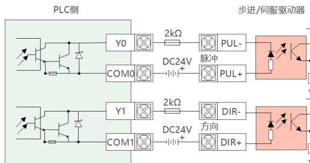
图 3-4 高速脉冲输出接线
