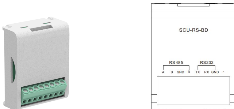
图 5-6 产品外观及端子定义
