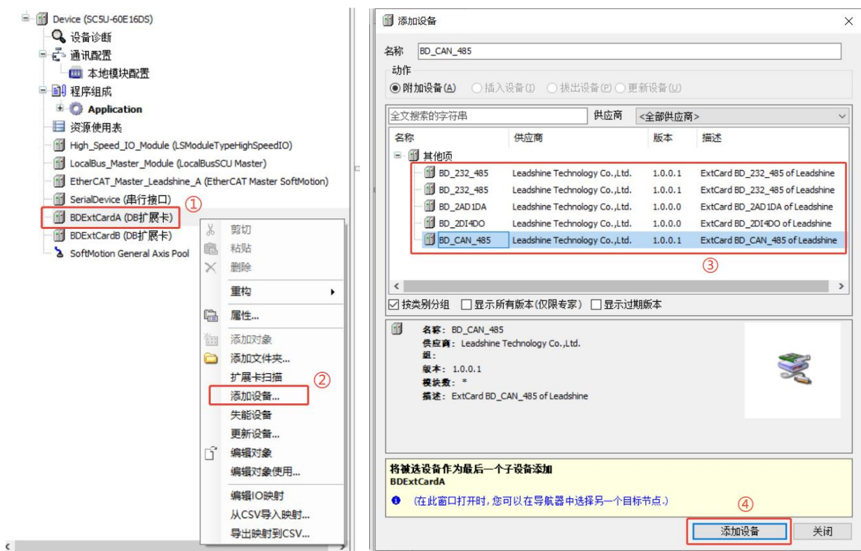
图 5-2 通过“添加设备”方式添加BD块
