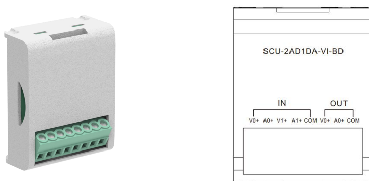
图 5-3 产品外观及端子定义
