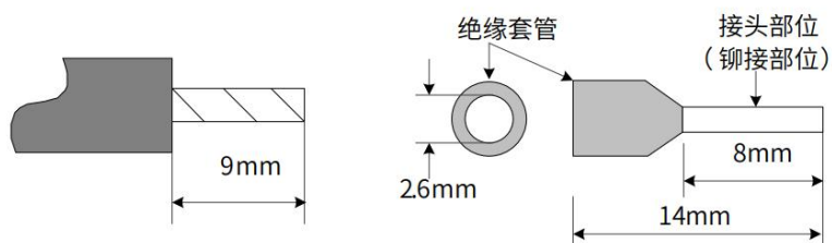
图 4-5 棒状端子接线
