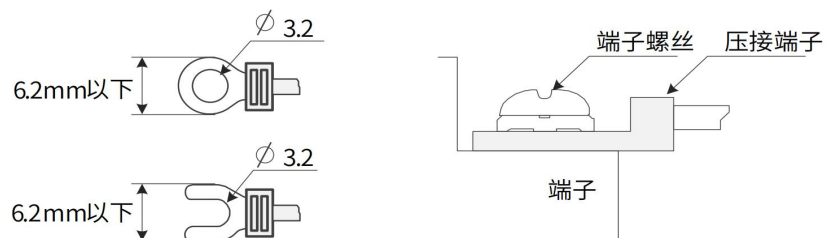
图 4-3 端子台接线端子
