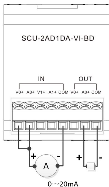
电流输入/输出接法
