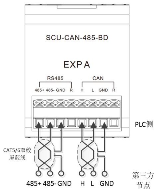
CAN/RS485通讯接法
