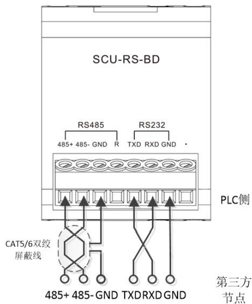
RS485/RS232通讯接法
