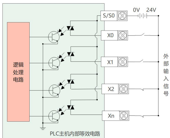
图 3-2 源型输入接线（PNP型传感器）
