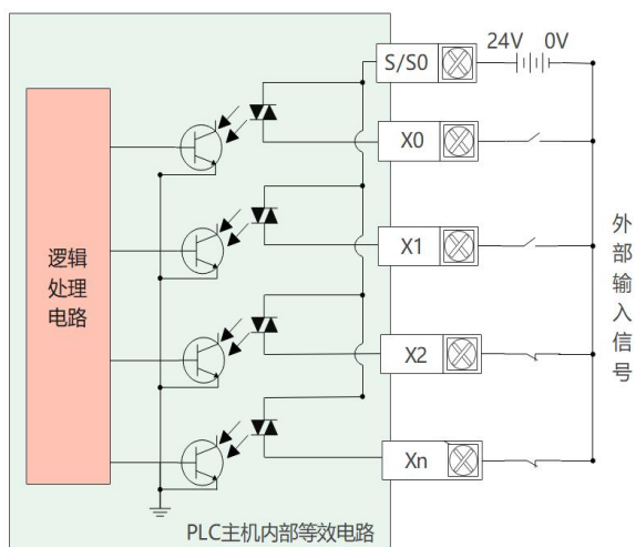
图 3-1 漏型输入接线（NPN型传感器）
