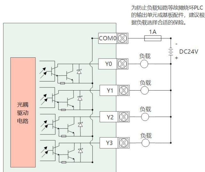
图 3-3 普通晶体管输出接线
