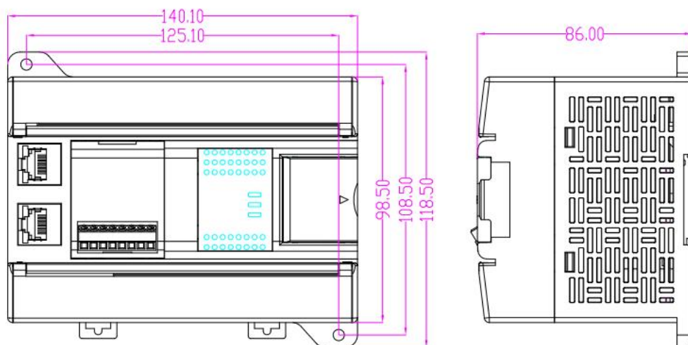
图 4-1 32和40点主机外观尺寸
