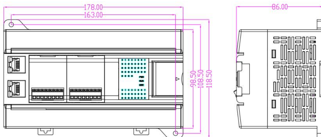
图 4-2 60点主机外观尺寸
