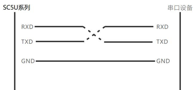
图 6-4 RS232总线通信连接
