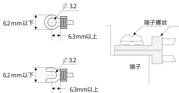
图 4-4 端子台接线端子
