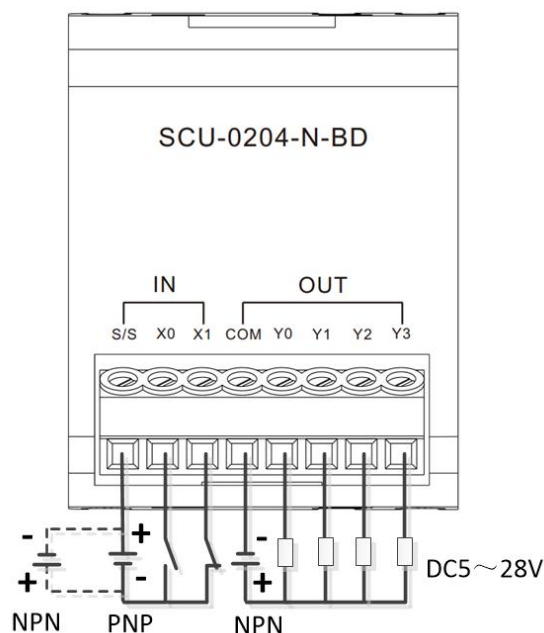
数字量输入/输出接法
