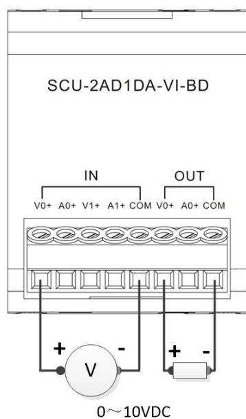
电压输入/输出接法
