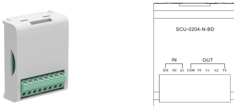
图 5-4 产品外观及端子定义
