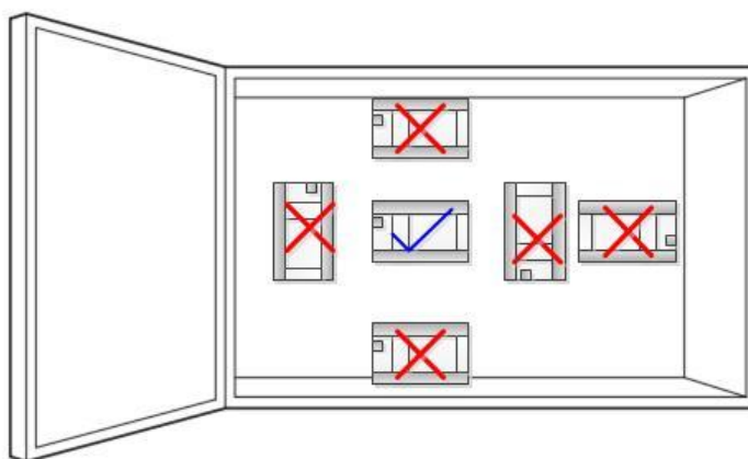
图 8-1 控制柜中PLC安装方式
