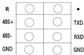
图 6-2 RS485 & RS232通信端口示意
